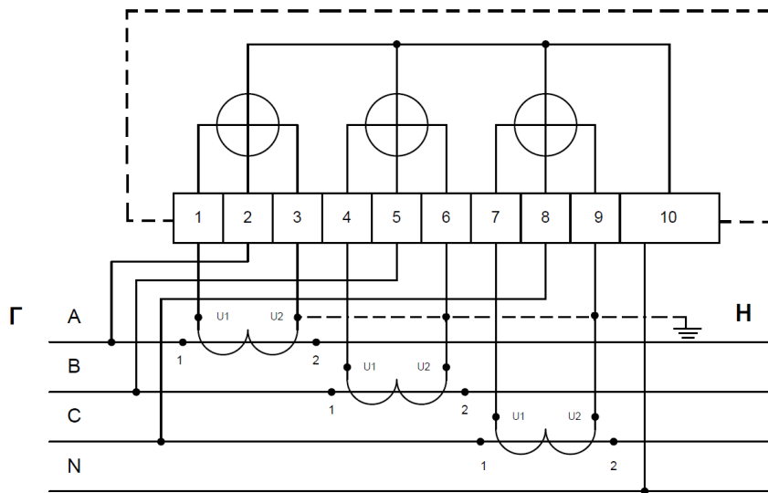
Схема підключення лічильника з номінальною напругою 3x220/380В, 3x230/400В та 3x240/416В
