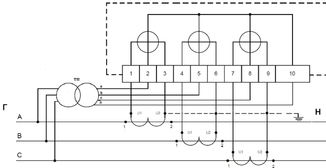
Схема підключення лічильника з номінальною напругою 3x57.7/100В
