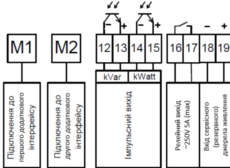
Рисунок 2 – Схема підключення інтерфейсів лічильника
