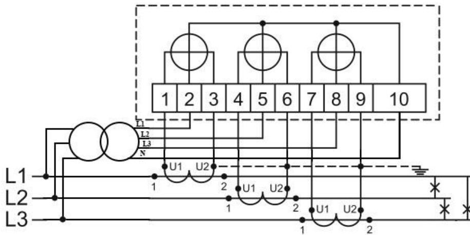
Схема підключення лічильника з номінальною напругою 3x57.7/100В
