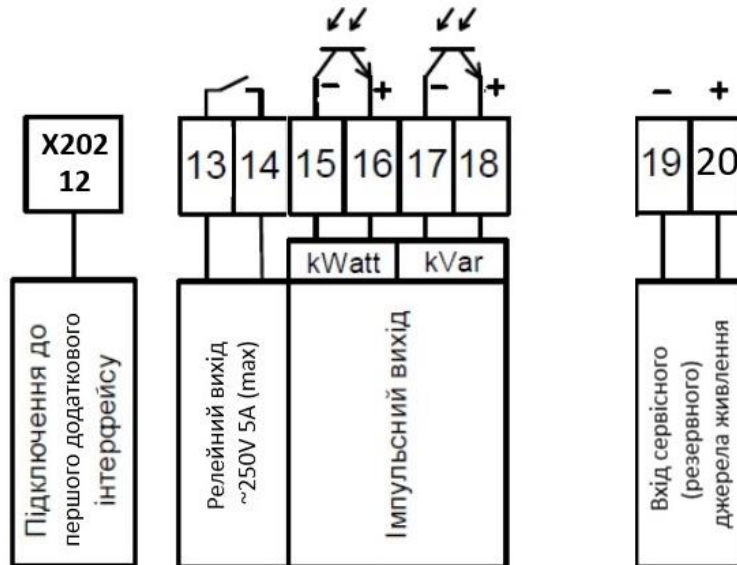
Рисунок 2 – Схема підключення інтерфейсів лічильника
