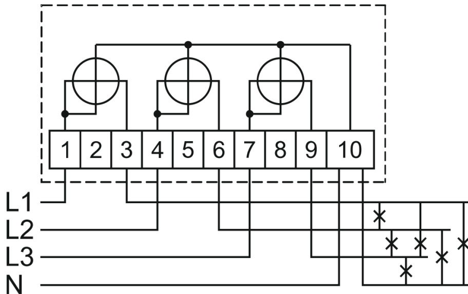
Рисунок 1 - Схема підключення лічильника до мережі споживача
