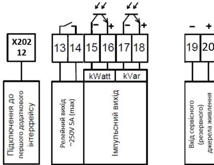
Рисунок 2 – Схема підключення інтерфейсів лічильника
