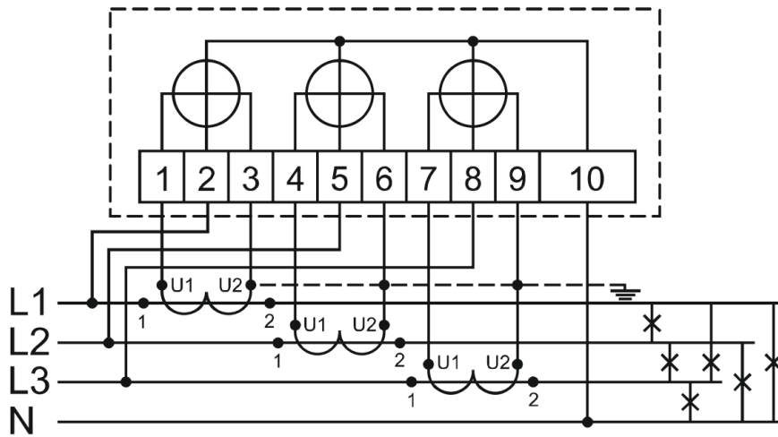
Схема підключення лічильника з номінальною напругою 3x220/380В, 3x230/400В та 3x240/416В
