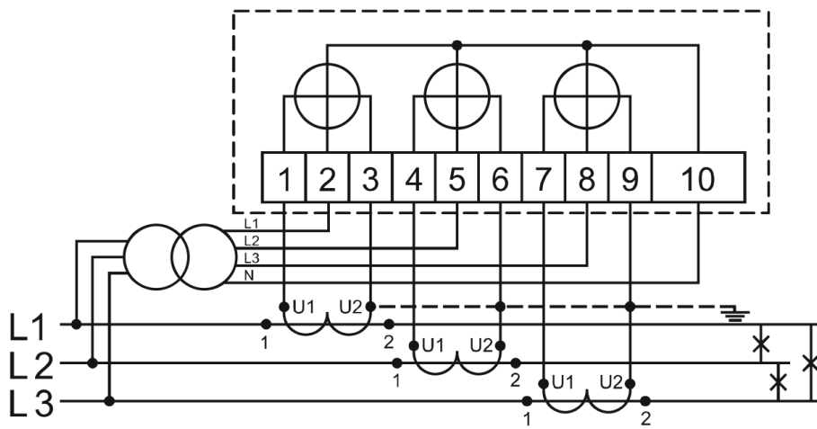
Схема підключення лічильника з номінальною напругою 3x57.7/100В
